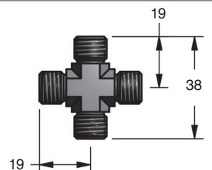
90.508.501 (D-501) Raccordo a Croce
