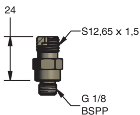
90.805.115 Raccordo Adattatore per fori di attacco - Dritto
