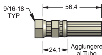
90.504.743 (S-743) Raccordo Tubo Compatto
