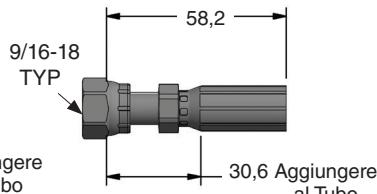
90.504.451 (SK-451) Raccordo Tubo Retraibile
