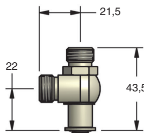
90.505.438 (S-438) Raccordo Adattatore
