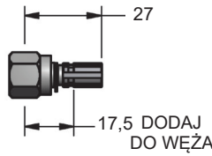
90.508.943 (D-943) Kompaktywny Obracać
