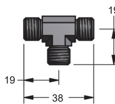
90.508.401 (D-401) Trójkąt
