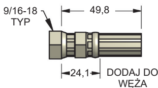
90.504.843 .SS (S-843) Kompaktowy Obracać
