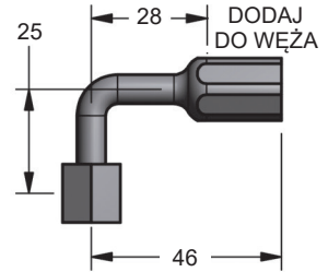
90.508.858 (D-858) 90° Obracać
