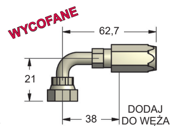
90.504.659 (S-659) 90° Obracać (dla Y-250)
