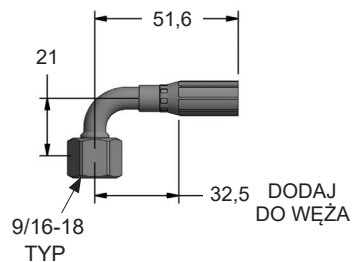
90.504.559 (SK-559) 90° Obracać
