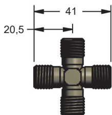
90.806.501 Krzyż
