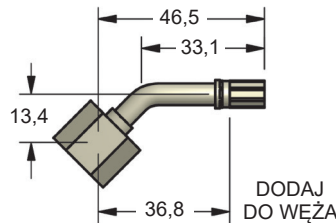
90.504.954 (S-954) 45° Obracać
