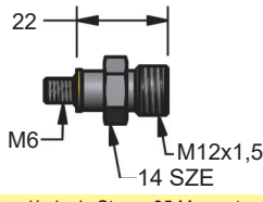
90.508.116 (D-116) Prosto
