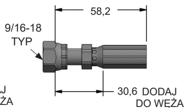
90.504.451 (SK-451) Chowany Obracać
