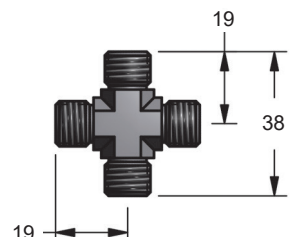
90.508.501 (D-501) Krzyż
