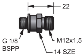
90.508.115 (D-115) Prosto
